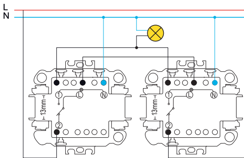
Váltókapcsolás ellenőrzőfényrel
