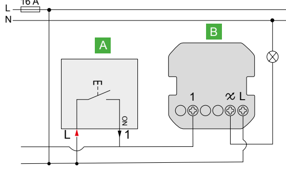
Egypólusú nyomó
