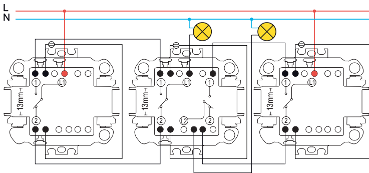
Kettős váltókapcsolás
