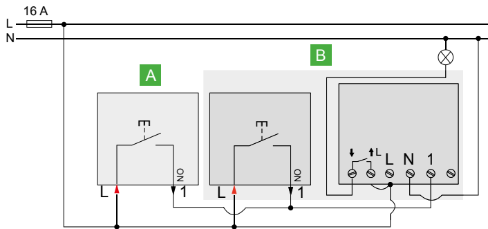
Egypólusú nyomó
