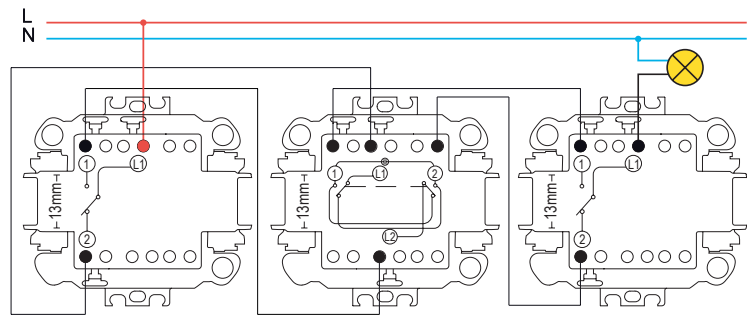
Keresztkapcsolás (jelzőfényrel vagy anélkül)
