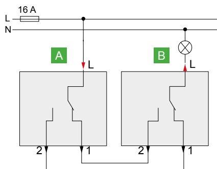
Váltókapcsoló
