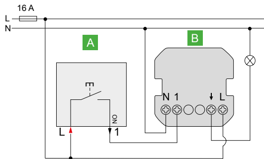
Egypólusú nyomó
