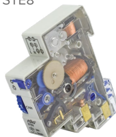
Lépcsőházi automata STE8 Time relay STE8
