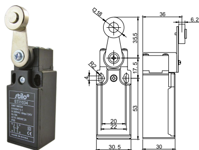
STI 1034 - Karos-görgős végálláskapcsoló Roller arm type
