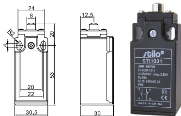
STI 1031 - Bütőkös végálláskapcsoló Push plunger type
