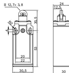
STI1032 - Görgős végálláskapcsoló / Roller plunger type
