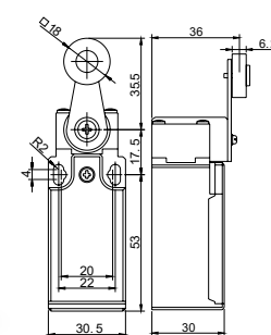
STI1034 - Karos-görgős végálláskapcsoló / Roller arm type
