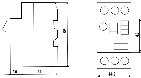
Méret / Size (mm)
