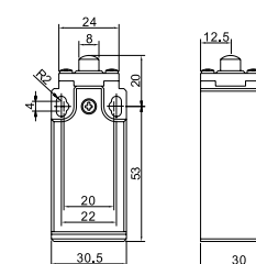
STI1031 - Büttykös végálláskapcsoló / Push plunger type
