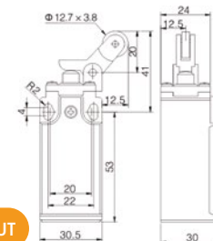
STI1381 - Egyirányú, függőleges működtetésű görgős végálláskapcsoló / Vertical roller lever type
