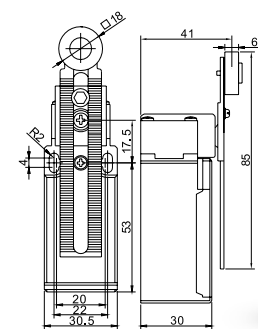
STI1035 - Állítható karos-görgős végálláskapcsoló / Adjustable roller arm type
