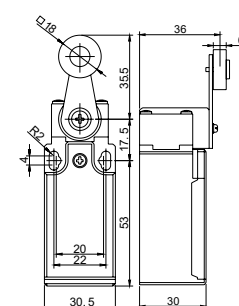
STI 1034 - Karos-görgős végálláskapcsoló Roller arm type
