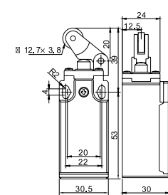
STI 1033 - Egyirányú vízszintes működtetésű görgős végálláskapcsoló / Horizontal roller lever type
