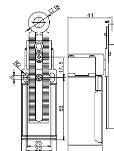
STI 1035 - Állítható karos-görgős végálláskapcsoló / Adjustable roller arm type
