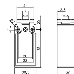
STI 1031 - Büttykös végálláskapcsoló Push plunger type
