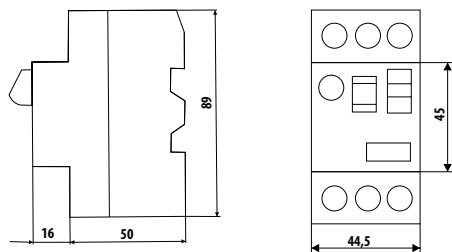
Méretek / Size (mm)
